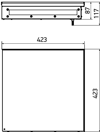
KVU 420-85-90
