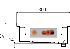
KVZs 300-105-xxxx.00.000
