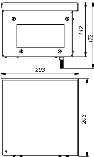
KVU 250-85-135
