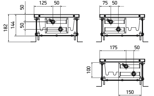
KVZ(KVP) 300-140
