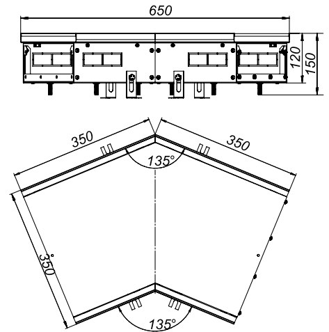
KVU 350-120-135
