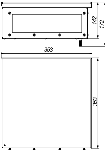
KVU 350-140-90
