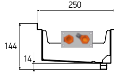
KVZs 250-120-xxxx.00.000
