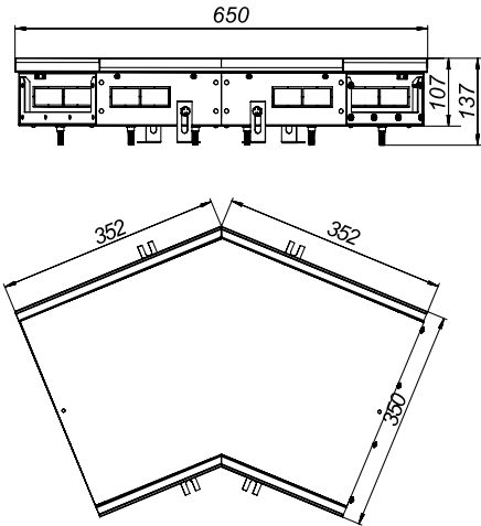
KVU 350-105-135
