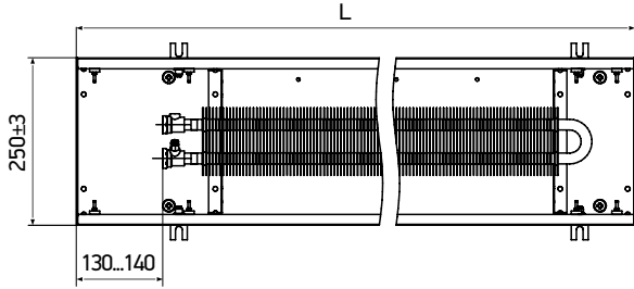
KVP 250-85 (105)
