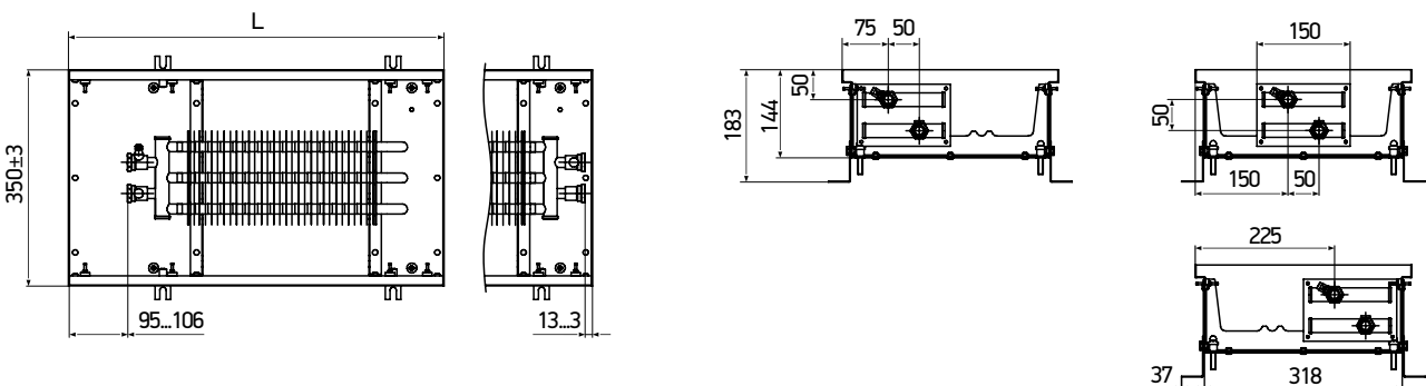
KVZ 350-140
