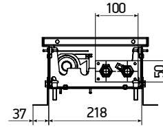
KVZV (KVPV) 250-140
