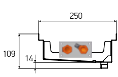
KVZs 250-85-xxxx.00.000
