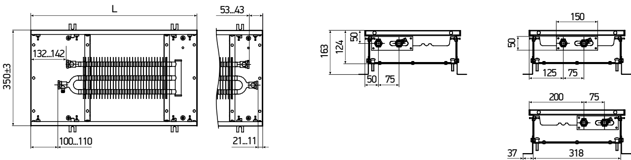
KVZ 350-120
