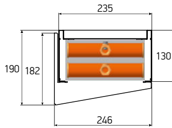
KPZ 235-130-xxxx.00.000-01/C
