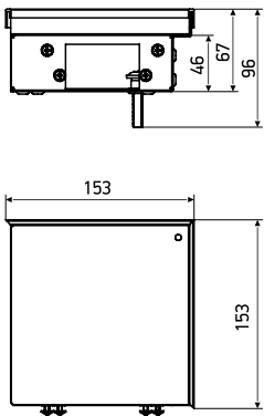
KVU 150-65-90
