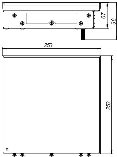
KVU 250-105-90
