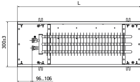
KVP 300-140
