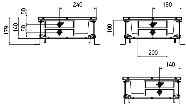
KVZ (KVP) 380-140
