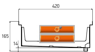
KVZs 420-140-xxxx.00.000
