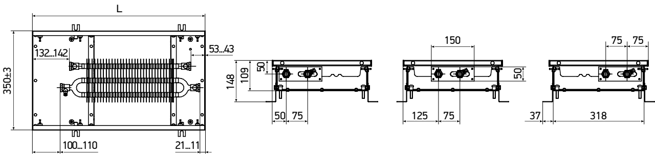
KVP 350-85 (105)
