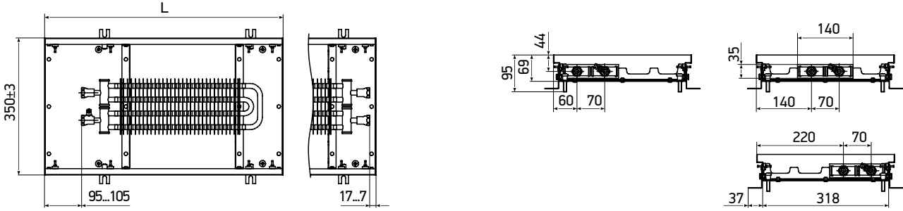
KVZ 350-65
