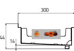
KVZs 300-120-xxxx.00.000
