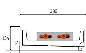
KVZs 380-105-xxxx.00.000
