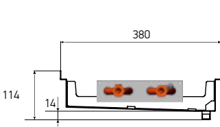
KVZs 380-85-xxxx.00.000
