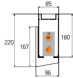
KPZ 85-180-xxxx.00.000-01/C
