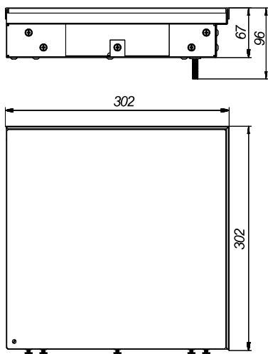
KVU 300-65-90
