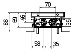
KVZ(P) 150-65
