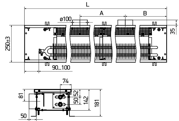
KVVZ 250-140
