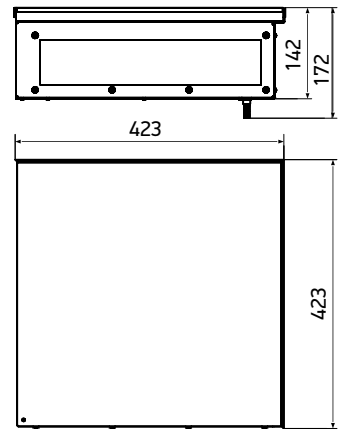
KVU 420-140-90
