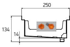
KVZs 250-105-xxxx.00.000
