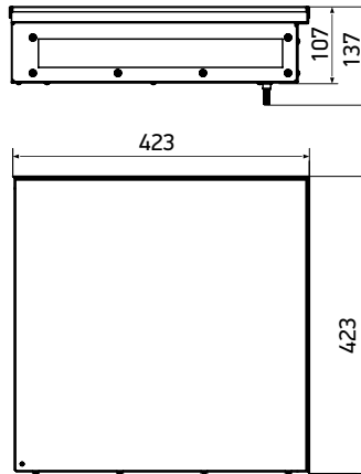
KVU 420-105-90
