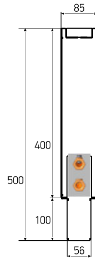
KPZ 85-400-xxxx.00.000-01-2
