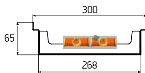
KVZ 300-85-xxxx.00.000
