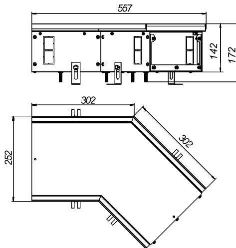
KVU 250-140-135
