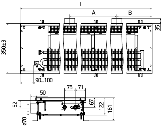
KVVZ 350-120
