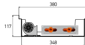
KVZV 380-120-xxxx.00.000
