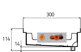
KVZs 300-85-xxxx.00.000
