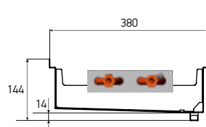
KVZs 380-120-xxxx.00.000
