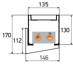
KPZ 135-130-xxxx.00.000-01-1/C
