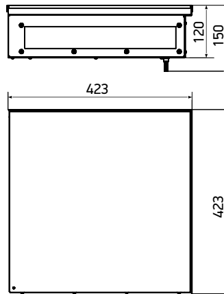
KVU 420-120-90
