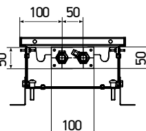
KVZ (KVP) 250-120
