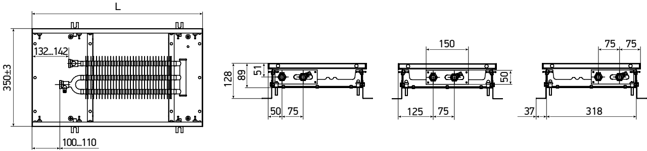
KVZ 350-85 (105)
