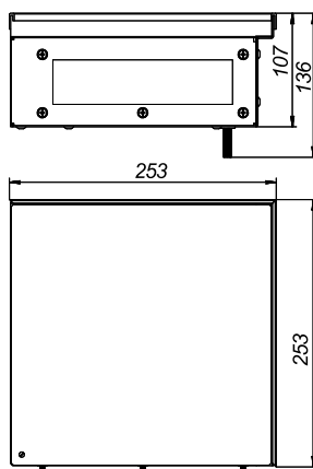
KVU 250-105-90
