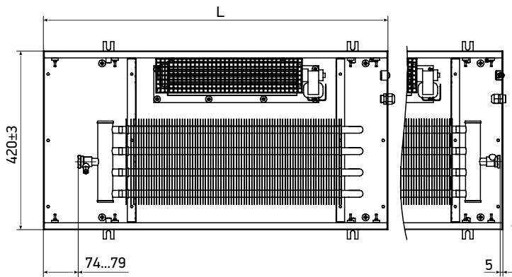
KVZV 420-140
