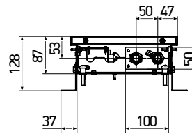
KVZV (KVPV) 250-85
