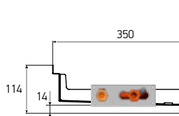
KVZs 350-85-xxxx.00.000
