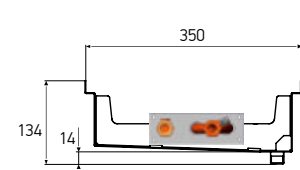
KVZs 350-105-xxxx.00.000
