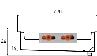
KVZs 420-120-xxxx.00.000
