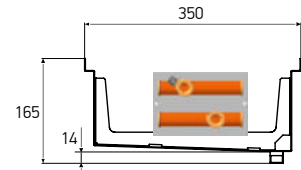
KVZs 350-140-xxxx.00.000
